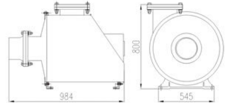
Blower B-2000LN
